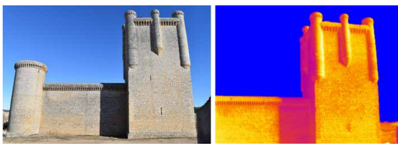
Confronto tra l'immagine nel visibile e l'immagine termografica di una delle superfici del Castello di Torrelobatón
